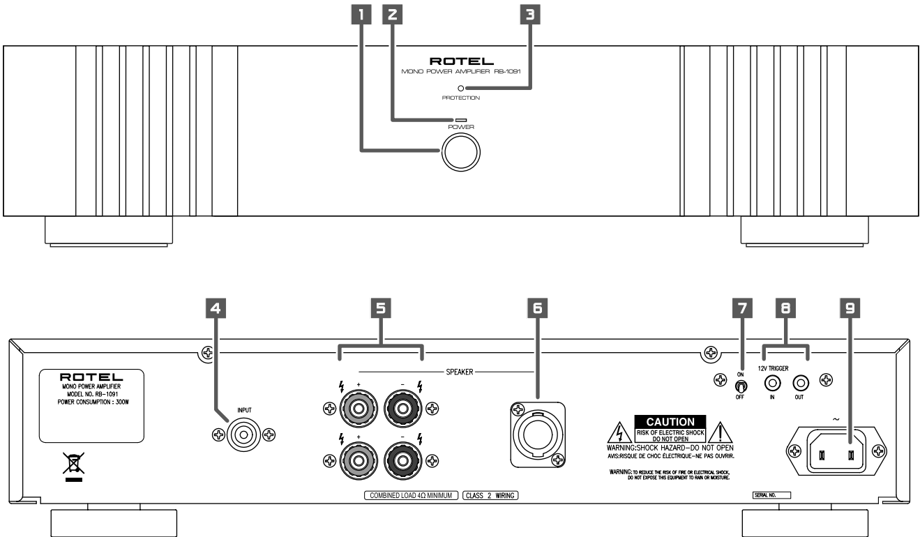
Figure 1: Controls and Connections Commandes et branchements Bedienelemente und Anschlüsse Pannello frontale e posteriore Controles y Conexiones De bedieningsorganen en aansluitingen Kontroller och anslutningar Органы управления и разъемы для подсоединения
